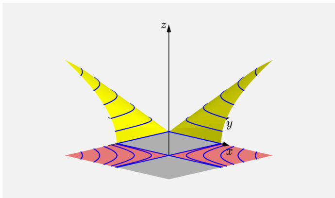
Obrázek 2: Vrstevnice funkce f(x, y)
